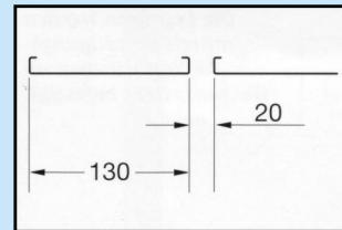
Abbildung: B-Profil
